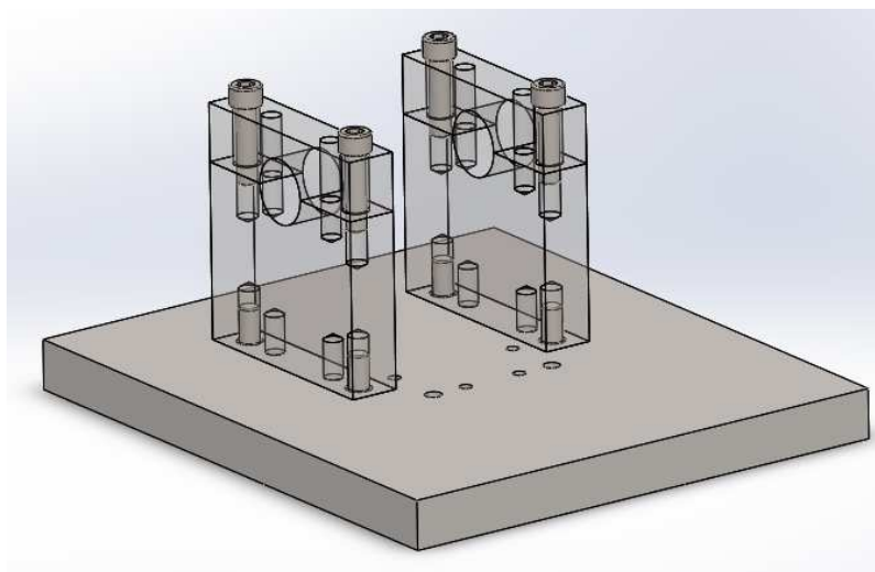
Slika 27: Dvodijelni oslonci za jednostavnije skidanje vratila
