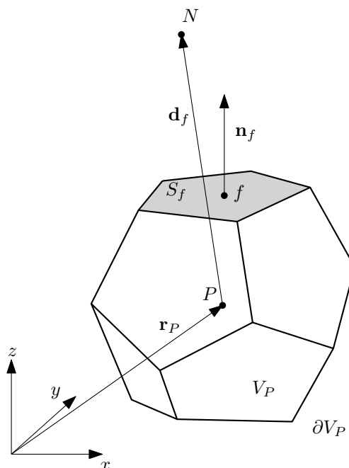
Slika 4.1: Kontrolni volumen
