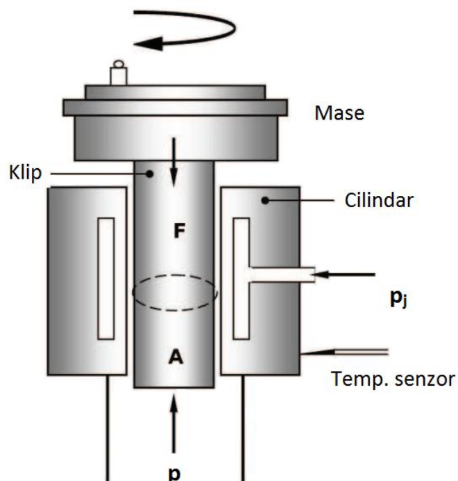
Slika 3. Sklop klip/cilindar
