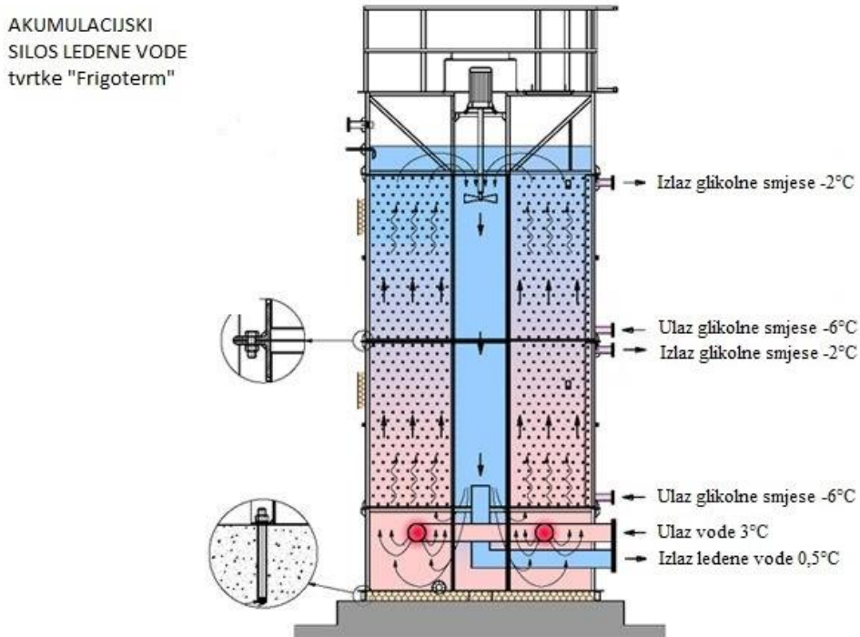
Slika 8. Shematski prikaz akumulacijskog silosa
