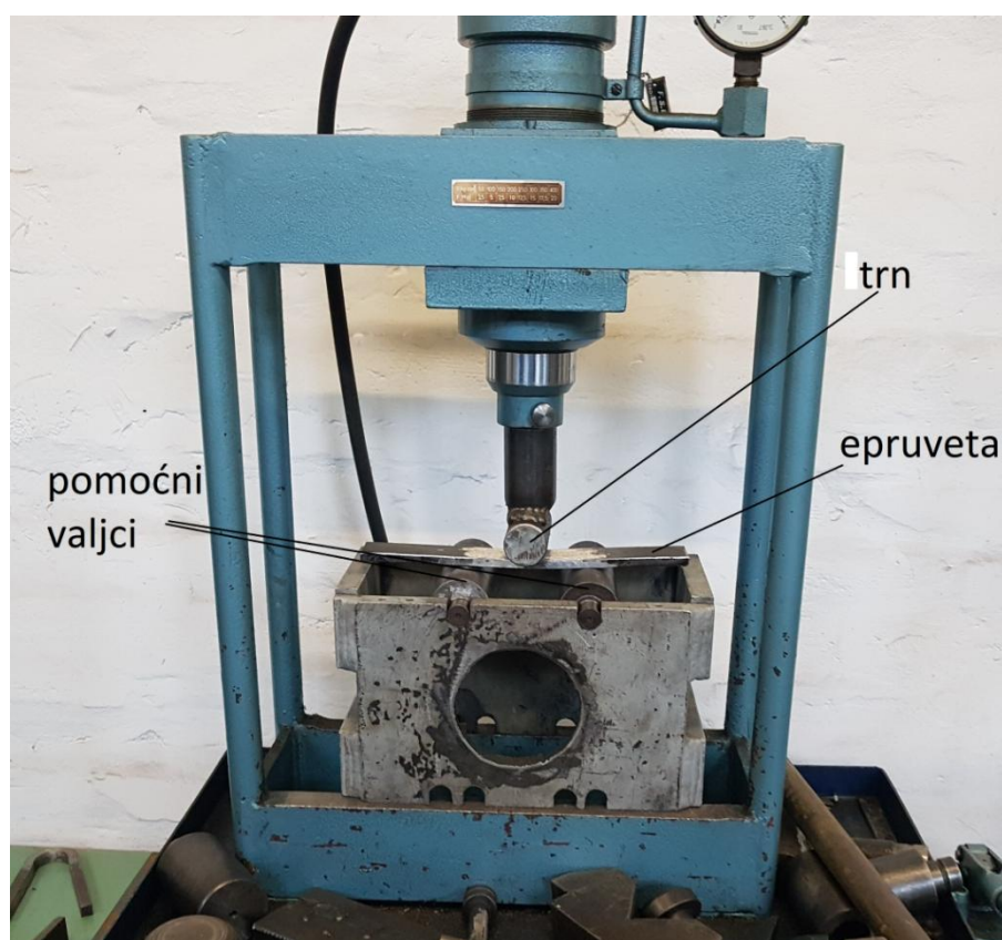
Slika 42. Naprava za ispitivanje savijanjem
