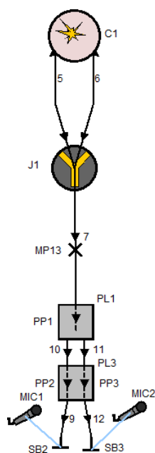
Slika 51. Simulacijski model s Akrapovičevim prigušivačem
