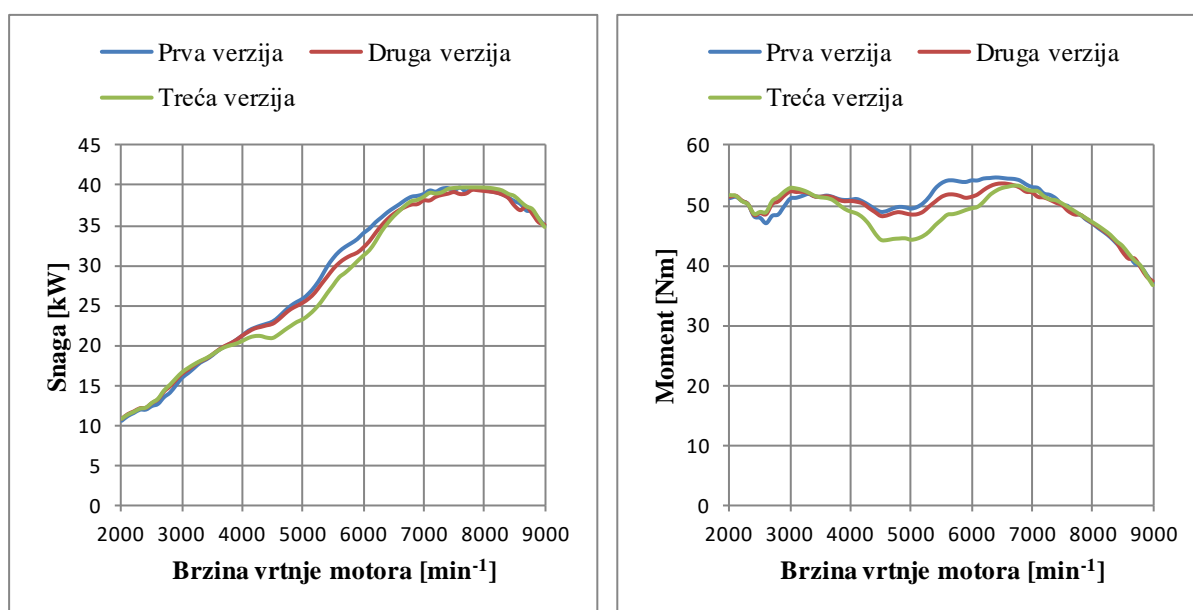
Slika 56. Usporedba performansi za slučajeve s dodatnim ispušnim cijevima iz prigušivača
