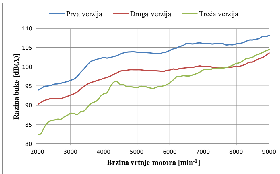
Slika 55. Usporedba razine buke za slučajeve s dodatnim ispušnim cijevima iz prigušivača
