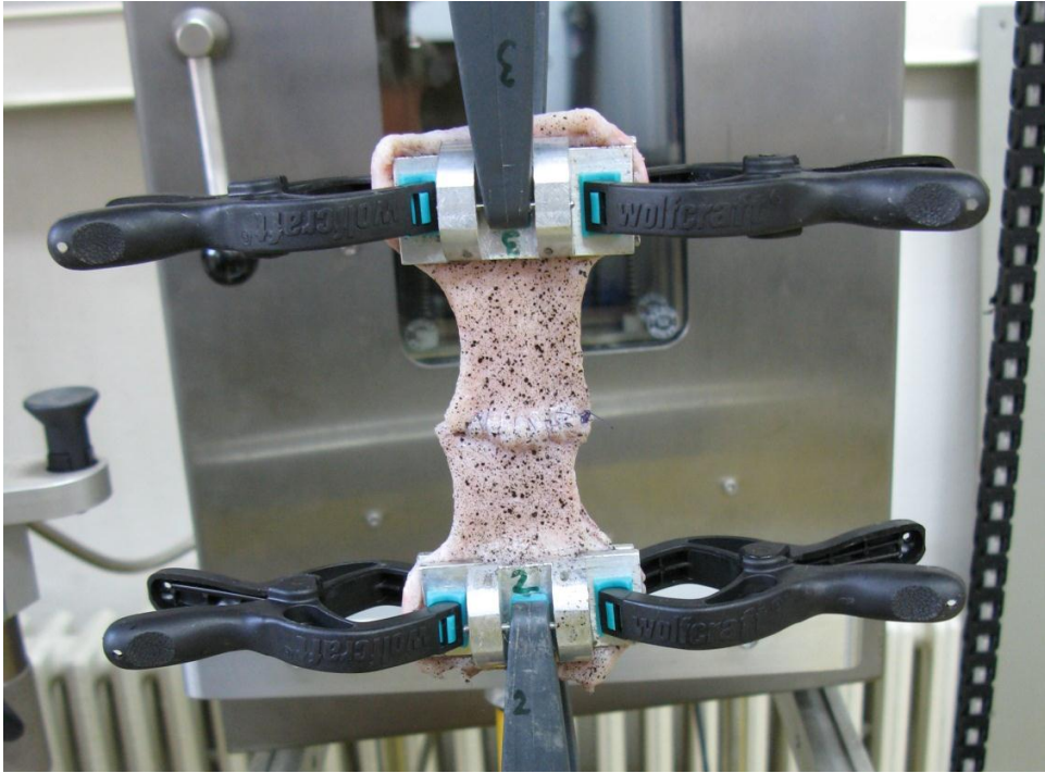
Slika 36 Uzorak učvršćen u prihvat kidalice
