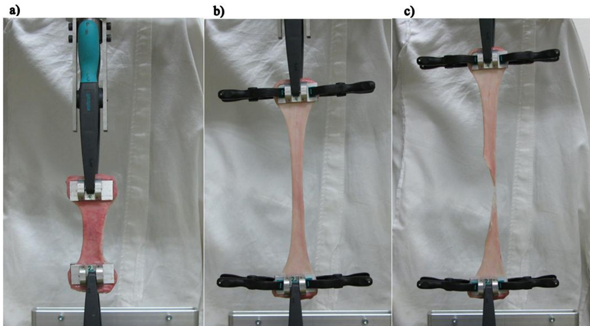
Slika 34 Vlačno ispitivanje uzoraka do pucanja: a) uzorak pozicioniran u prihvat, b) uzorak tijekom opterećivanja i c) uzorak neposredno prije pucanja
