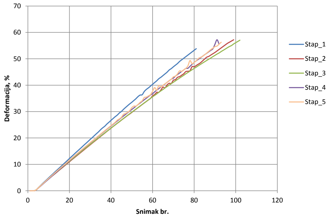
Slika 50 Dijagram deformacija za uzorke zatvorene staplerom
