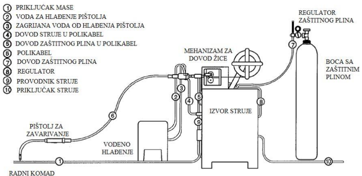
Slika 2. Oprema za MAG zavarivanje [4]
