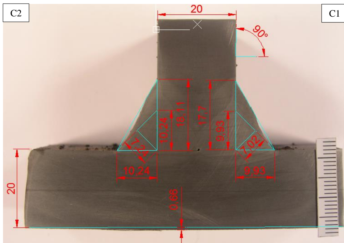
Slika 39. Prikaz standardnih dimenzija kutno zavara – uzorak C
