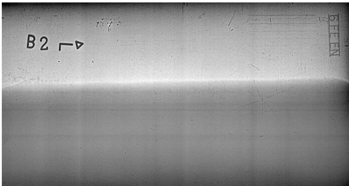
Slika 33. Radiogram zavara izveden konvecnionalnim Mag postupkom (strana B2)
