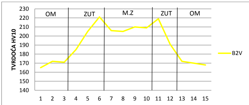
Slika 52. Prikaz tvrdoća na uzorku B2V
