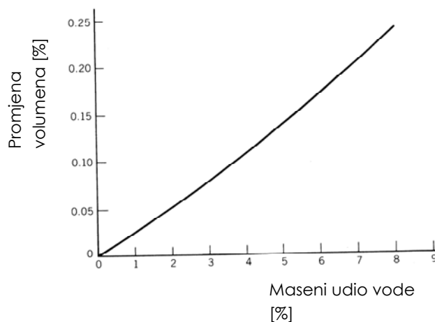
Slika 20. Promjena volumena uslijed apsorpcije vode poliamida 6[6]
