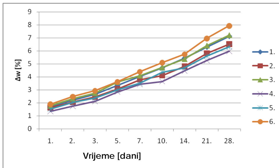
Slika 33. Apsorpcija vode epruveta PA 6
