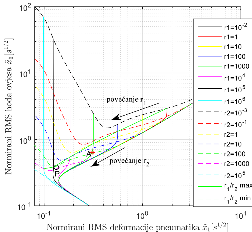
Slika 16. Kompromis između hoda ovjesa i deformacije pnematika za model s dva stupnja slobode gibanja
