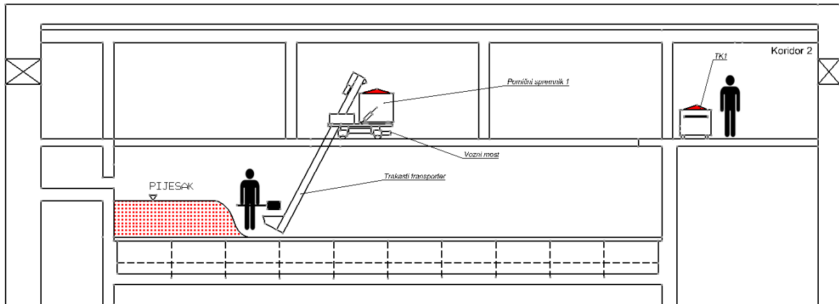
Slika 6.11 Koncept 7
