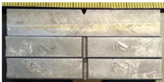
Slika 24. Charpy epruvete
