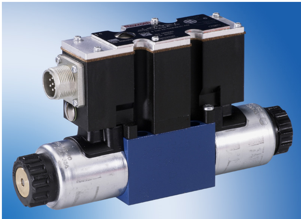
Slika 2.4: Proporcionalni razvodnik
