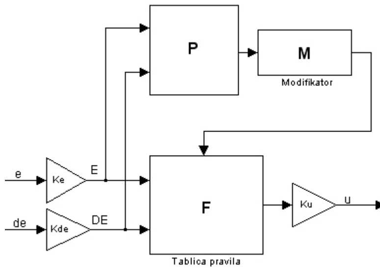
Slika 6.1: Struktura SONR-a
