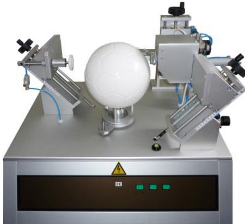
Slika 25. Uređaj za mjerenje radijusa [4]
