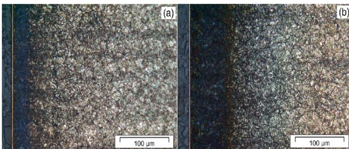
Slika 16 Poprečni presjek uzorka: a) TiBN5, b) TiBN80 [21]
