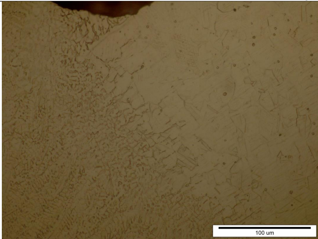
Slika 42. Mikrostruktura ZUT-a korijena zavara
