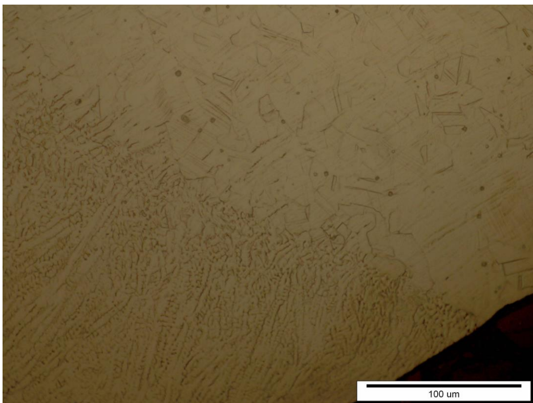
Slika 43. Mikrostruktura ZUT-a tjemena zavara
