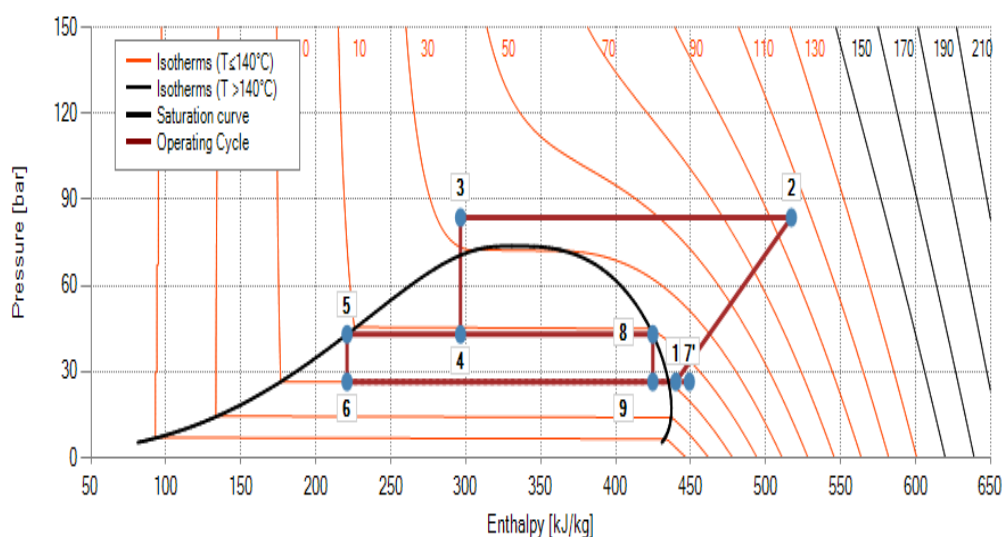
Slika 8. p,h dijagram za proces s ekspanzijskim ventilom u obilaznom vodu
