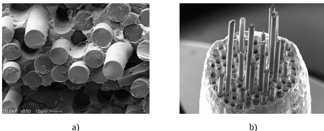
Slika 3. Mikrostruktura CMC i MMC kompozita: a) CMC - keramička matrica (SiC) ojačana SiC vlaknima [13]; b) MMC - metalna matrica (Cu) ojačana SiC vlaknima [14]
