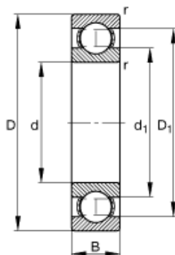
Slika 40. Dimenzije ležaja [9]
