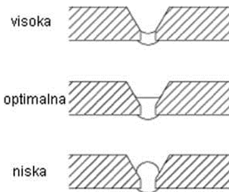
Slika 15. Utjecaj vršne struje na geometriju zavara [14]
