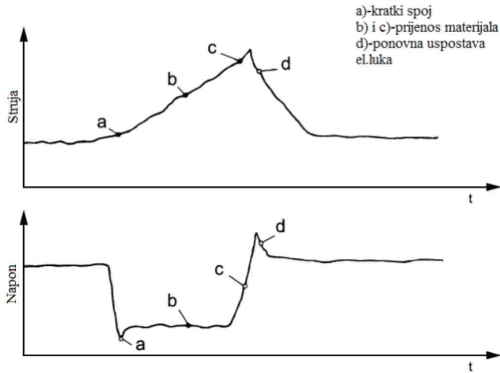
Slika 24. Faze EWM forceArc postupka zavarivanja [10]
