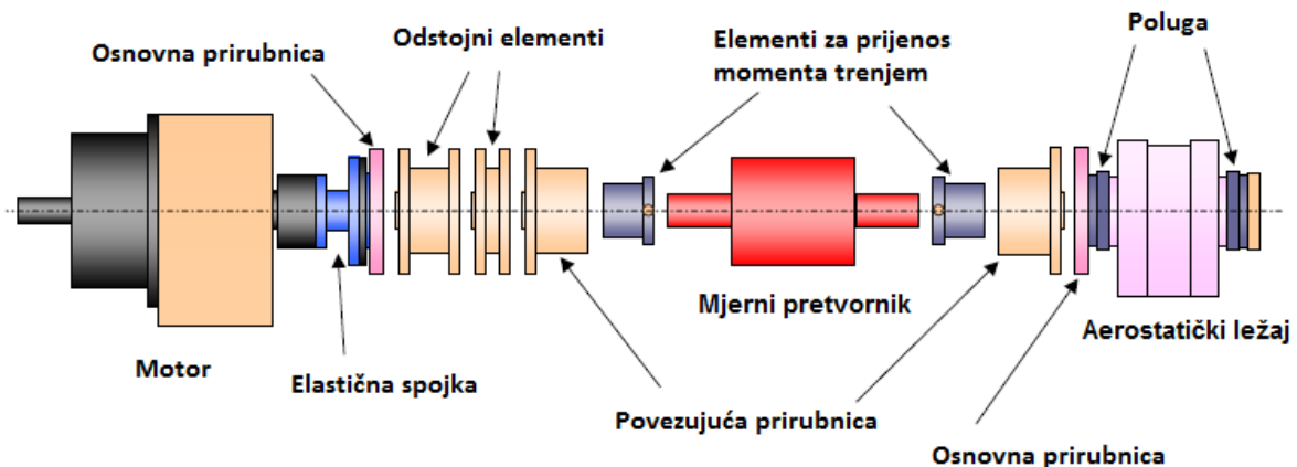
Slika 8. Shema za umjeravanje apsolutnom metodom (2) [6]
