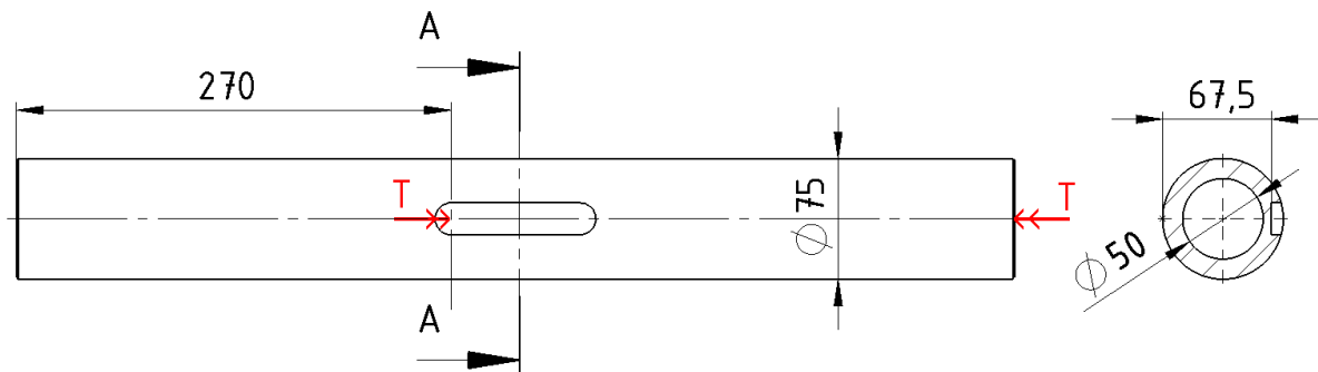
Slika 44. Vratilo s torzijskim opterećenjem
