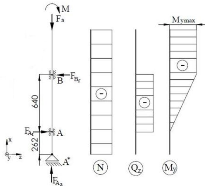
Slika 50. Dijagrami opterećenja osovine okretišta
