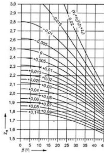
Slika 54. Dijagram faktora oblika boka [18]
