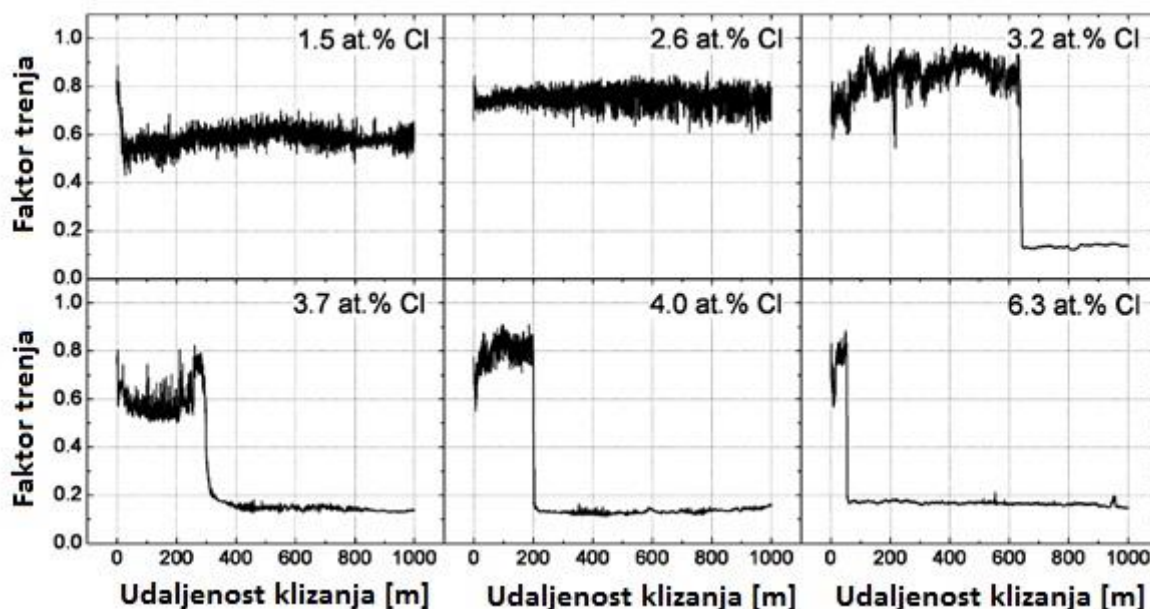
Slika 3.5 Snižanje vrijednosti faktora trenja TiN prevlake povećanjem koncentracije klora [10]
