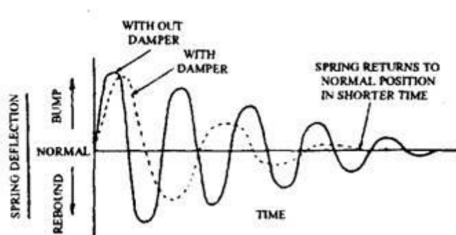
Slika 11. Prigušenje ovjesa [12]
