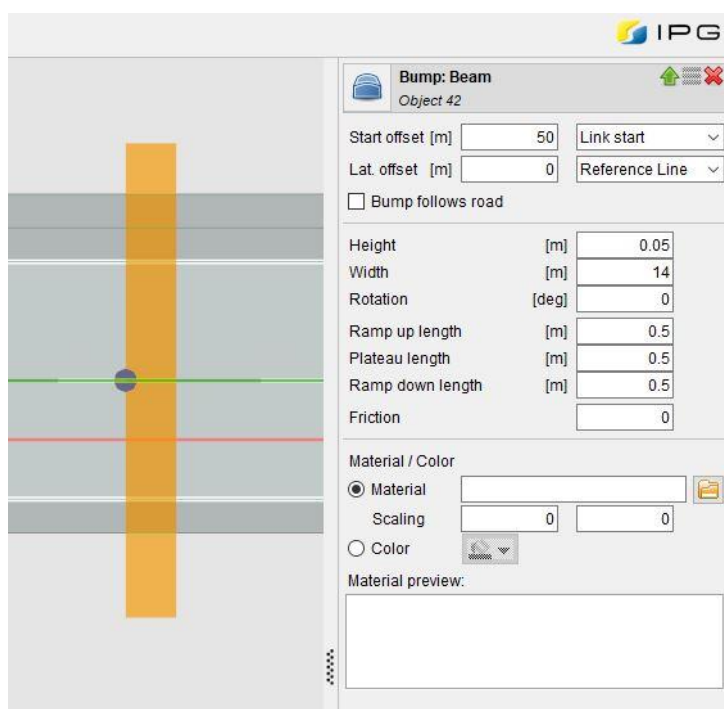
Slika 58. Parametri poprečne prepreke
