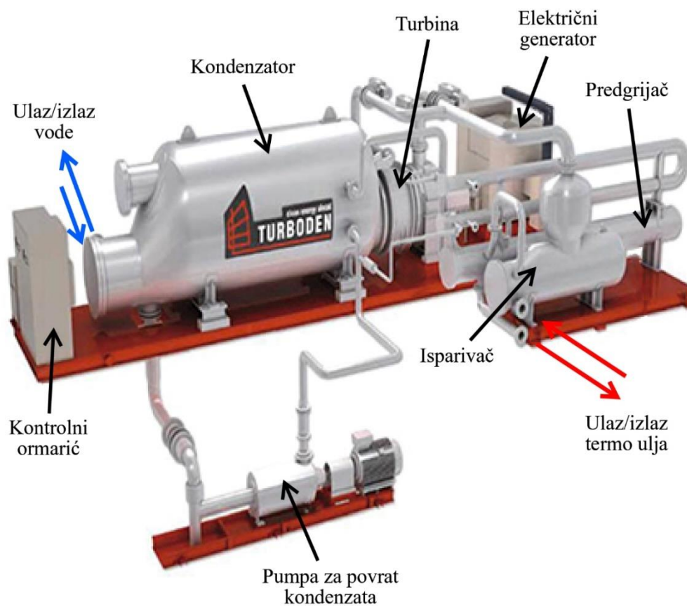
Slika 6. Turboden 10 CHP-Split [8]
