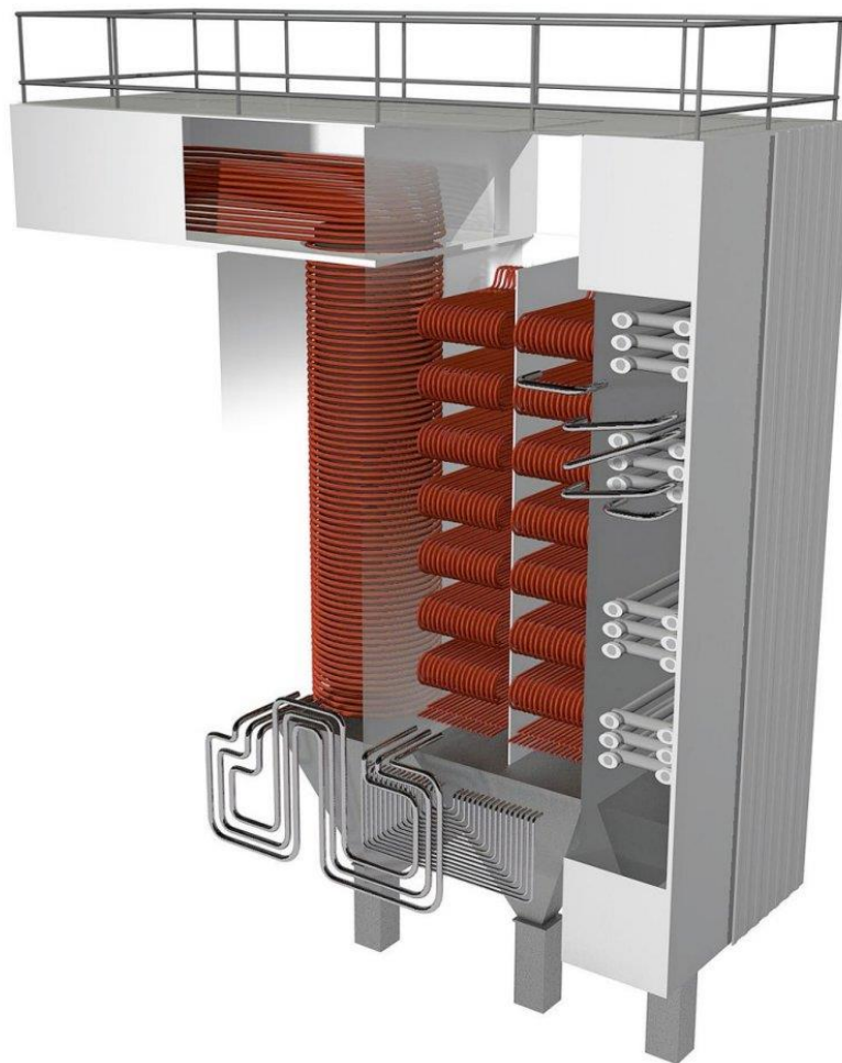
Slika 12. Termouljni kotao [16]
