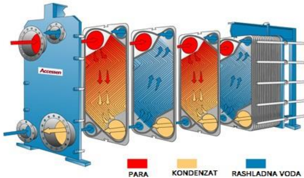
Slika 11. Pločasti kondenzator [6]
