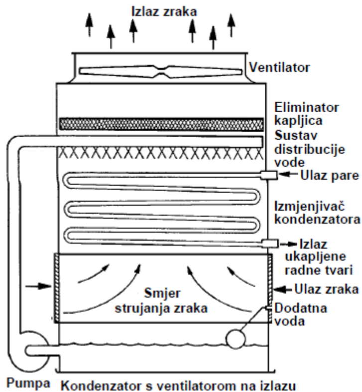
Slika 14. Evaporativni kondenzator [5]
