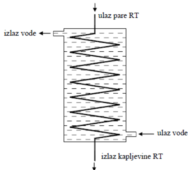
Slika 8. „Shell and coil“ kondenzator [2]
