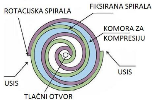
Slika 19. Presjek „scroll“ kompresora [8]
