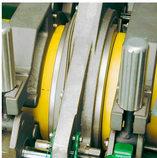
Slika 2. Struganje cijevi [7]
