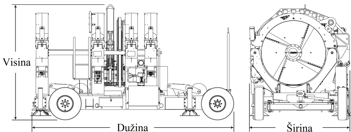
Slika 10. Dimenzije MegaMc 1600 [12]
