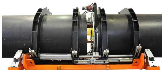
Slika 23. Delta 1600 Basic [24]
