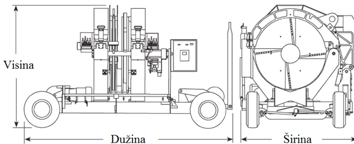
Slika 12. Dimenzije MegaMc® 2065 [13]
