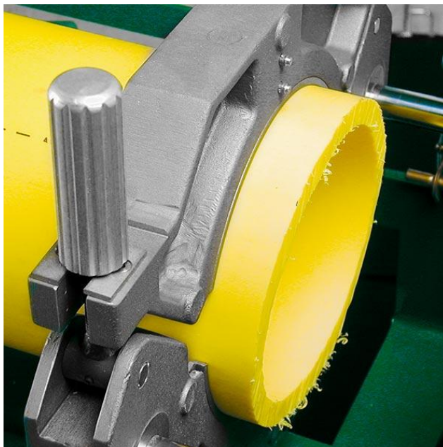
Slika 1. Stezanje cijevi [7]
