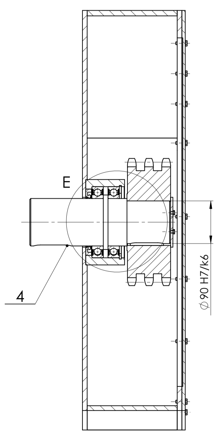
Presjek B-B
