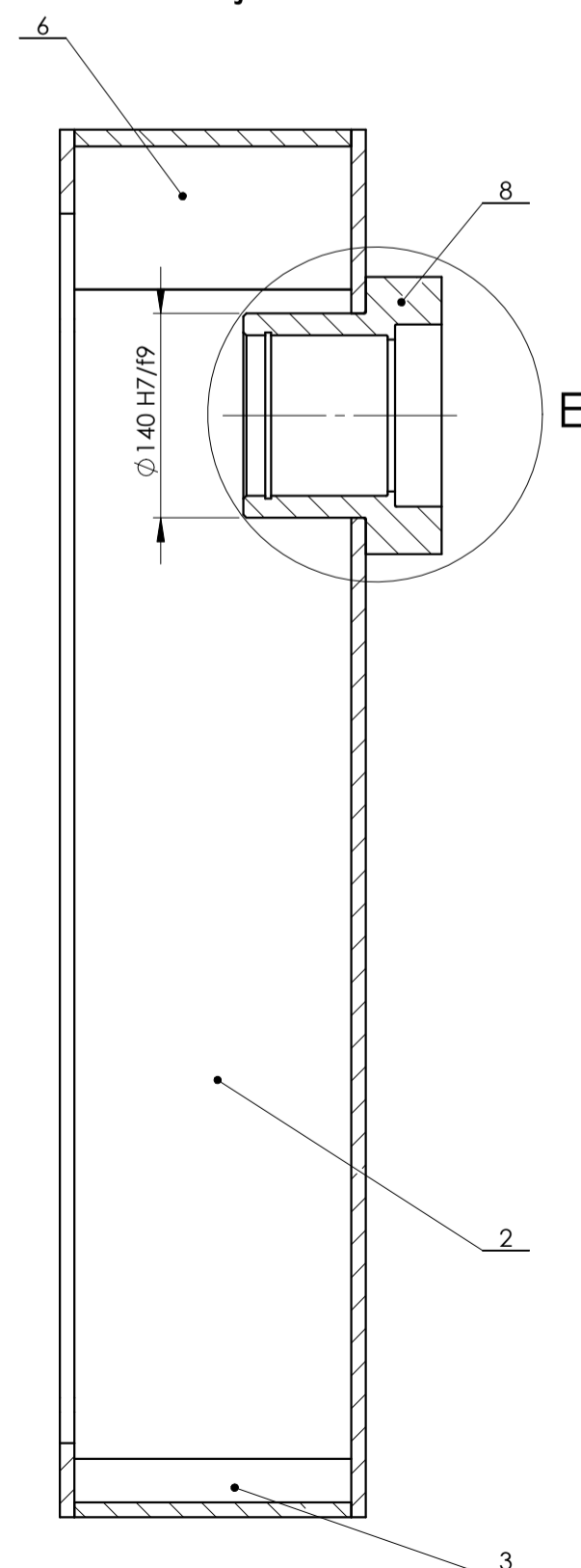
Presjek C-C
