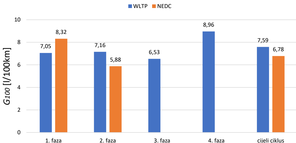
Slika 34. Prikaz rezultata potrošnje goriva po fazama WLTP i NEDC ispitnih ciklusa
