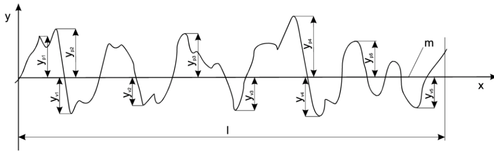
Slika 26. Parametar R_z
