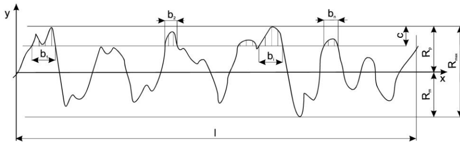
Slika 27. Parametar R_{max}
