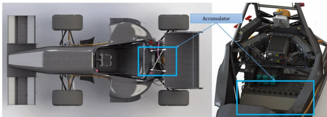
Slika 9. Pozicija baterijskog paketa
