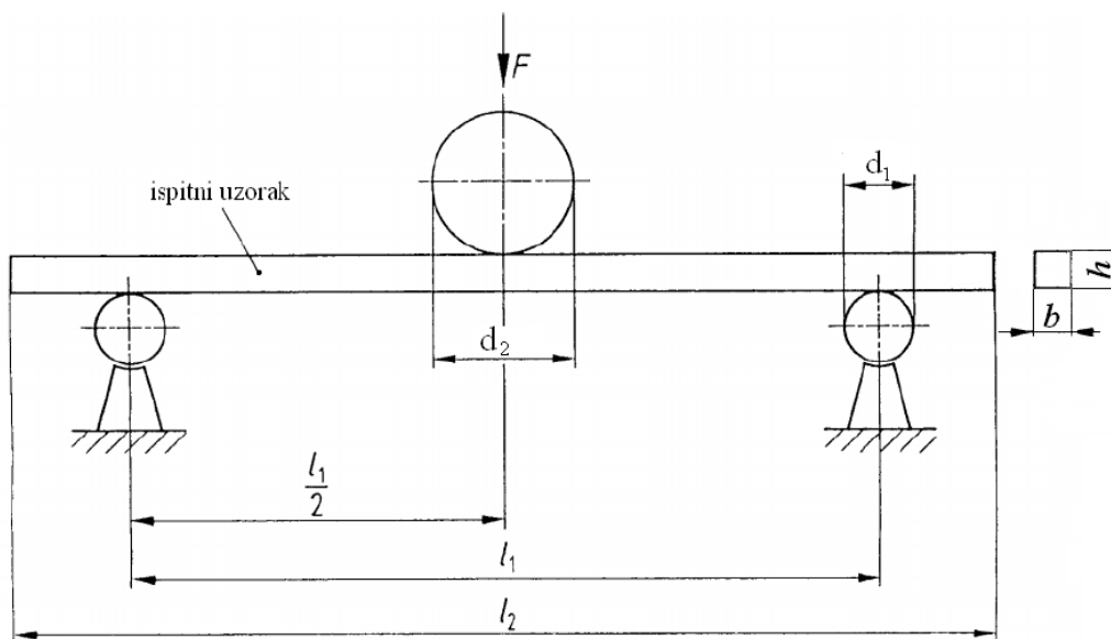
Slika 14. Postupak ispitivanja savojne čvrstoće [12]
