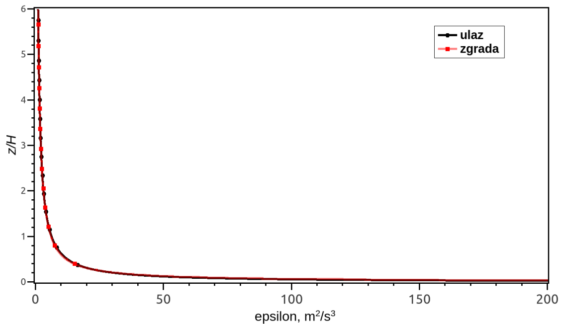
Slika 18. Usporedba profila disipacije kinetičke energije turbulencije \varepsilon(z) u 2D domeni sa suburbanim ulaznim profilom prema Kozmaru [18]
