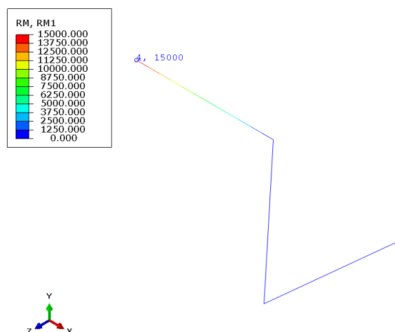
Slika 27. Prikaz reakcija veza, tj. momenata oko osi X u Nmm
