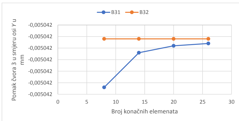
Slika 40. Konvergencija pomaka čvora 3 u smjeru osi Y u mm
