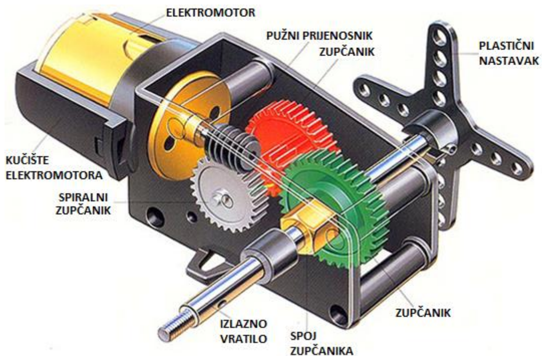
Slika 1. Unutrašnjost servomotora
