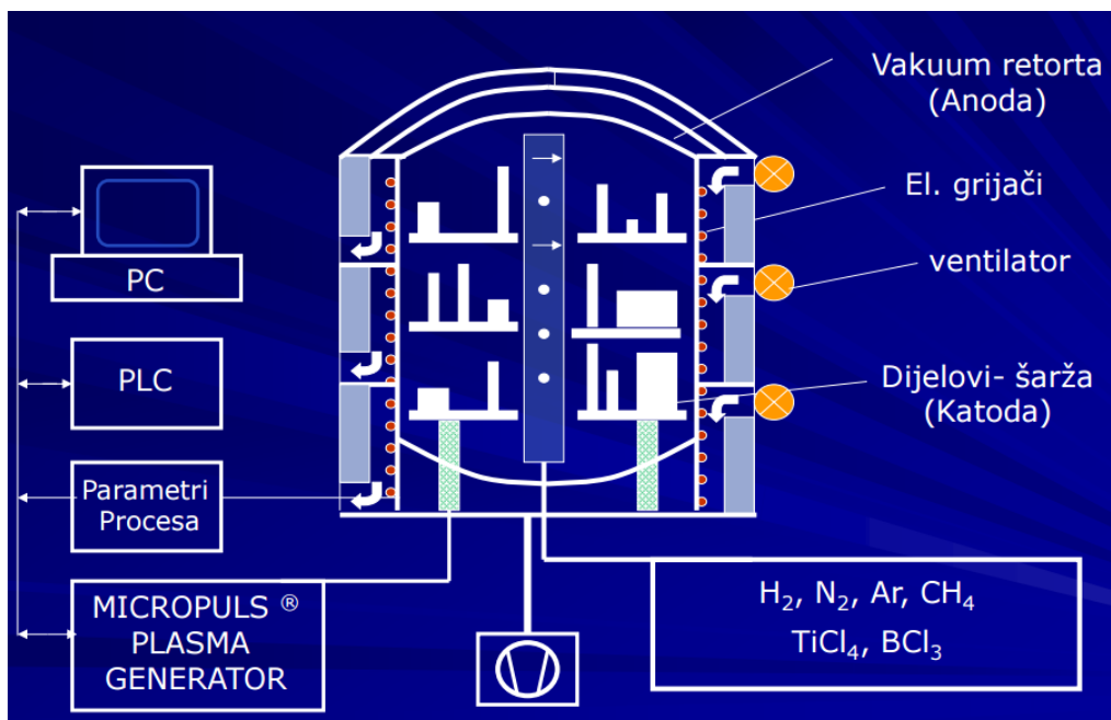
Slika 14. Shematski prikaz PACVD uređaja [6]
