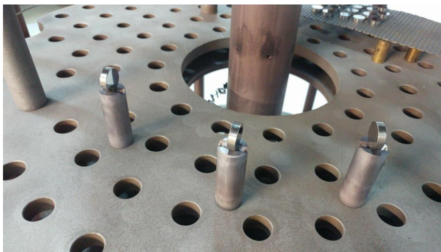
Slika 30. Položaj uzoraka za nitriranje u plazmi
