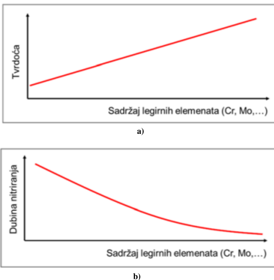
Slika 8. Utjecaj legirnih elemenata na: a) tvrdoću nitriranog sloja, b) dubinu nitriranog sloja[7]
