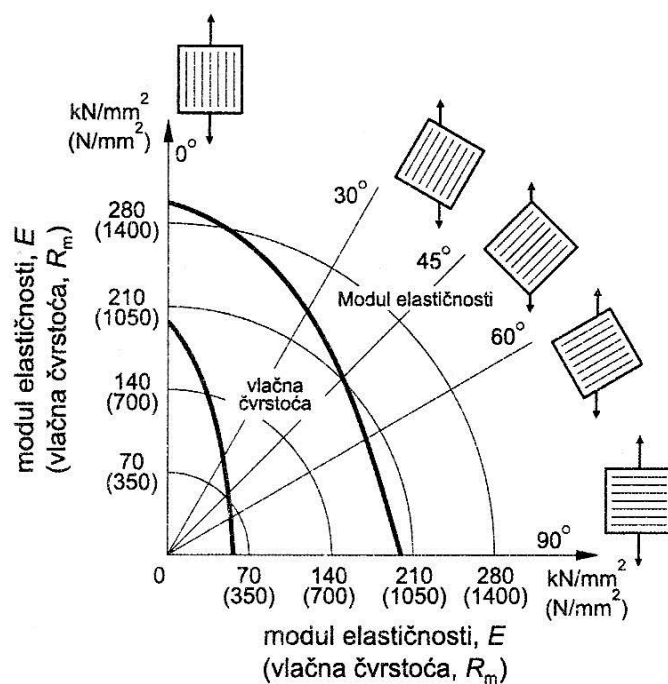
Slika 2.9 Usmjerenost vlakana [3]
