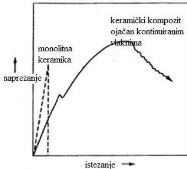
Slika 3.10 Dijagram naprezanje-istezanje monolitne keramike i CMC-a. [7]
