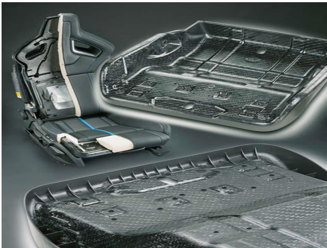
Slika 2.13 Sjedala iz Opel Insignije OPC [1]
