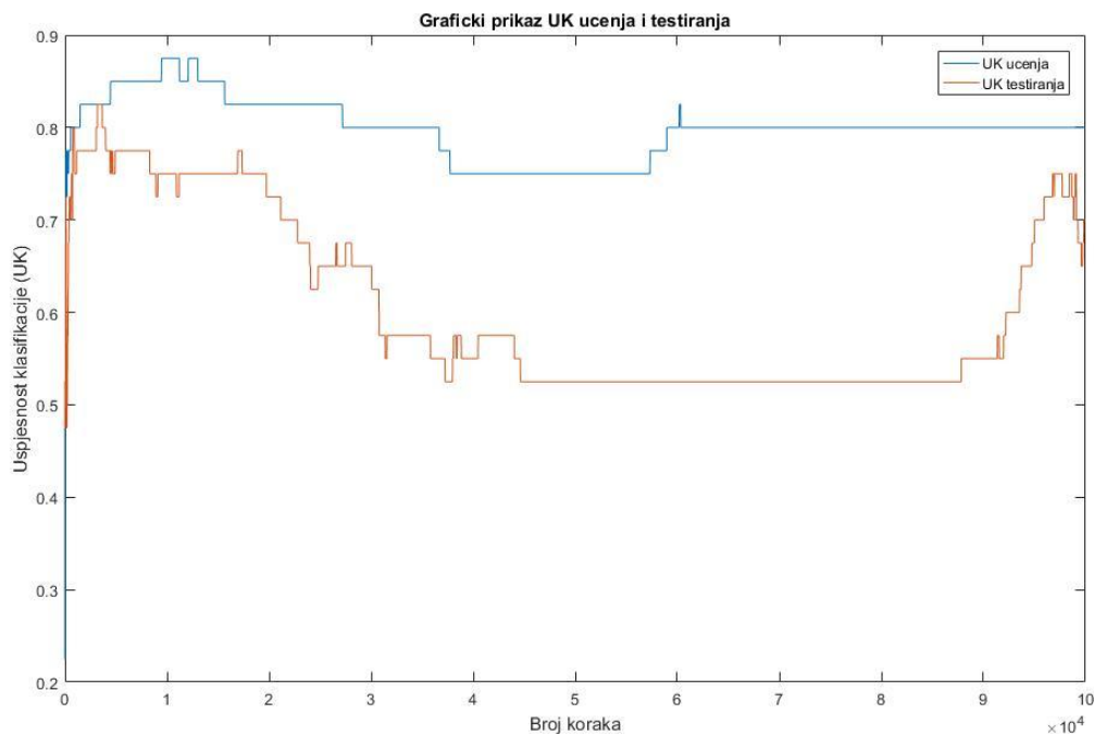
Slika 5.9. Grafički prikaz UK kod značajki struja pri \eta = 0.025 , \alpha = 0.01 , n_{skrivenih} = 3
