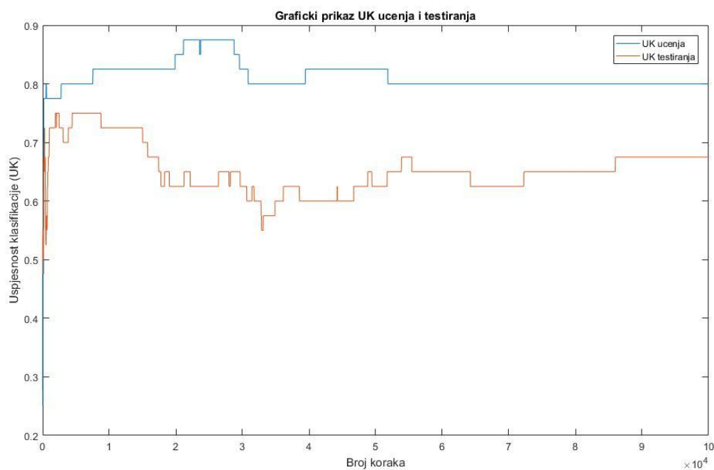
Slika 5.10. Grafički prikaz UK kod značajki struja pri \eta = 0.01 , \alpha = 0 , n_{skrivenih} = 3
