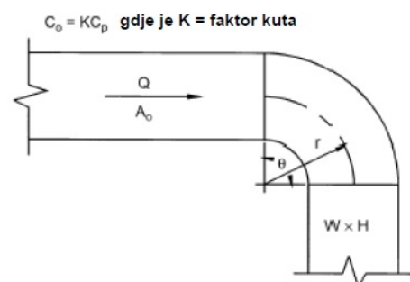
Slika 44 Tablica lokalnih gubitaka trenja za koljena
