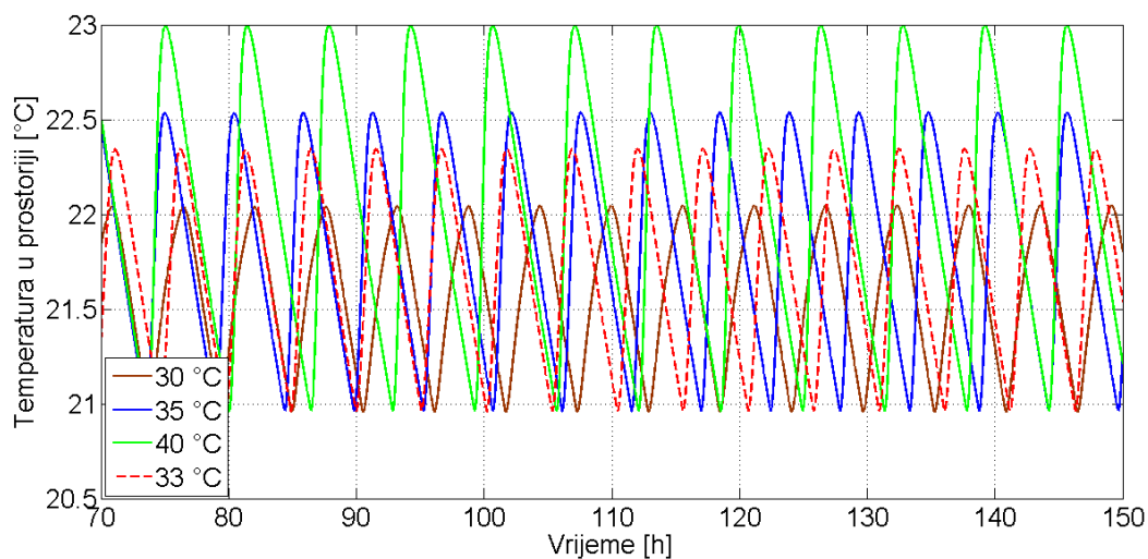
Dijagram 12. Odstupi temperature zraka pri promjeni temperature polaza
