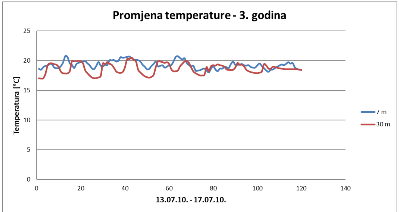
Graf 14: Promjena temperature u odabranom razdoblju u 2010. godini
