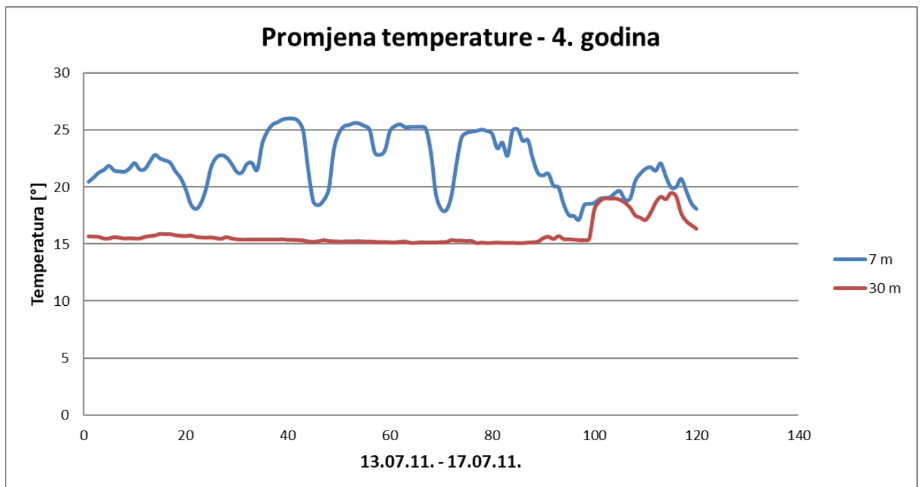
Graf 15: Promjena temperature u odabranom razdoblju u 2011. godini
