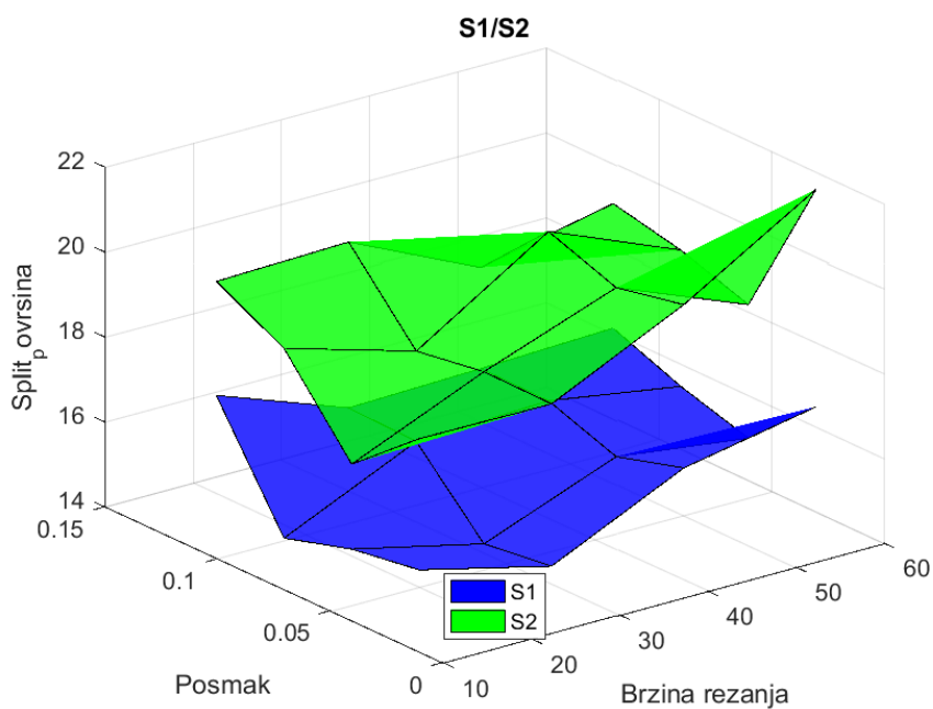
Slika 30. Srednji iznos delaminacije po korigiranim stupnjevima istrošenosti S1 i S2
