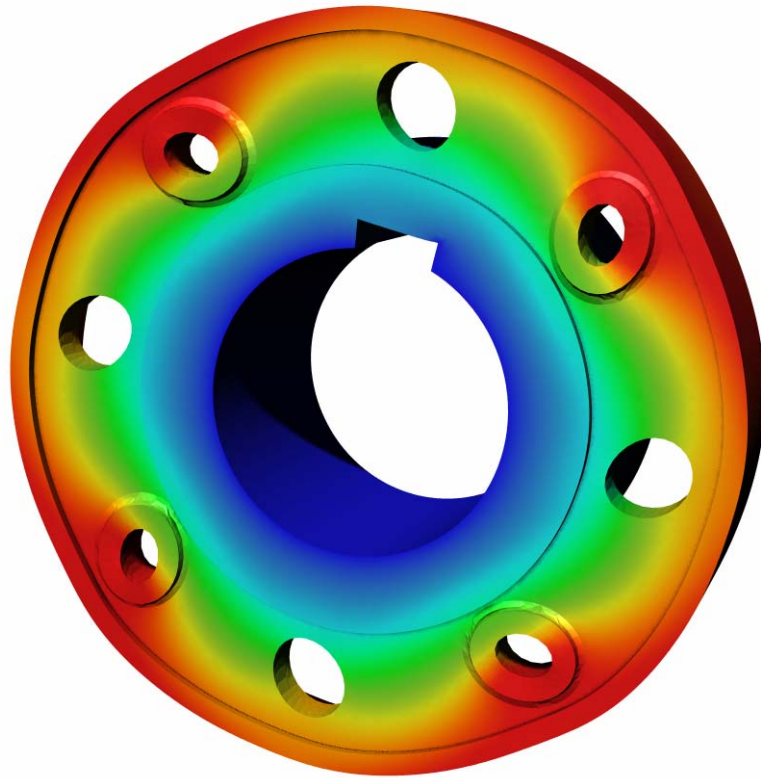
Slika 80. Deformirani oblik, deformacija je uvećana 2000 puta
