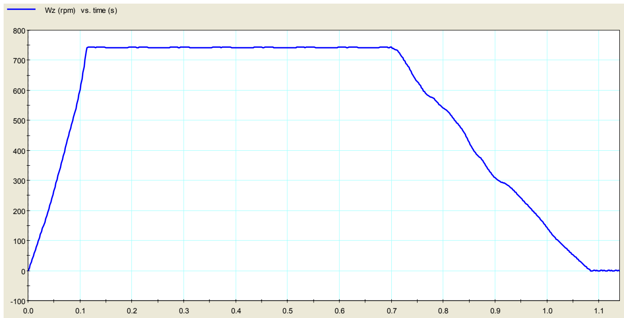
Slika 55. Dijagram brzine vrtnje rotora kompresora u ovisnosti o vremenu
