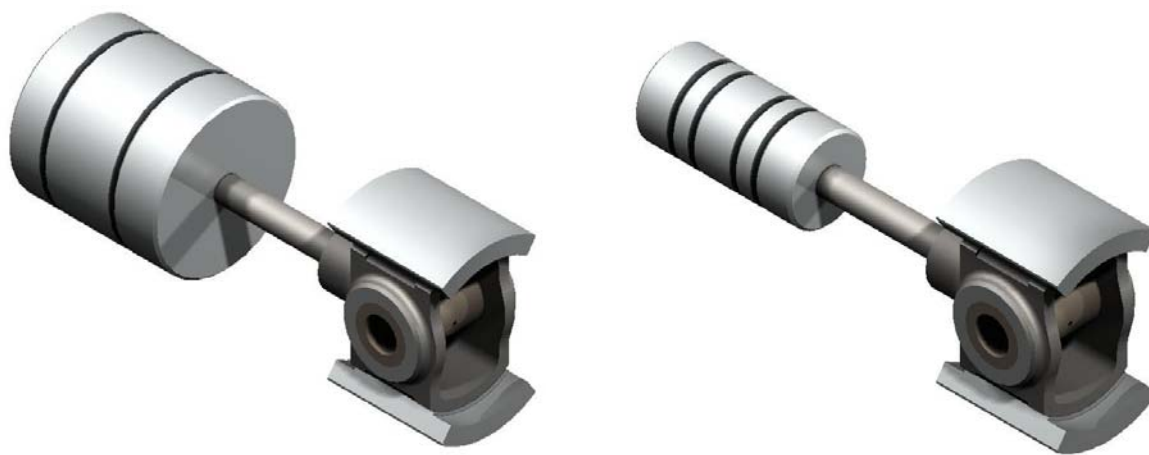
Slika 11. Križna glava i stap prvog stupnja (lijevo) i drugog stupnja (desno)
