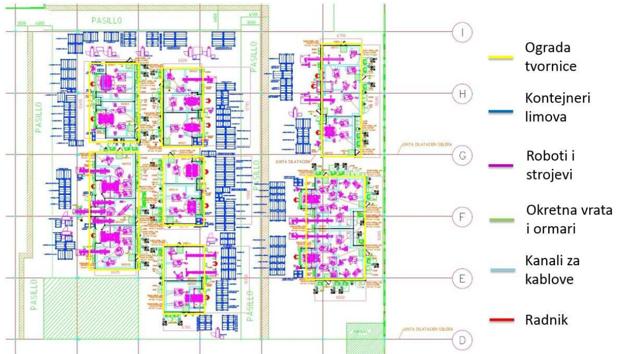
Slika 1. Shema dijela tvornice
