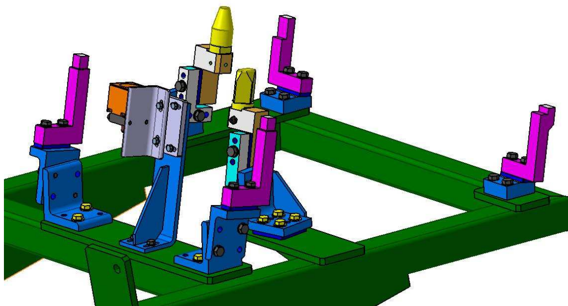
Slika 15. Pozicija reference u stroju
