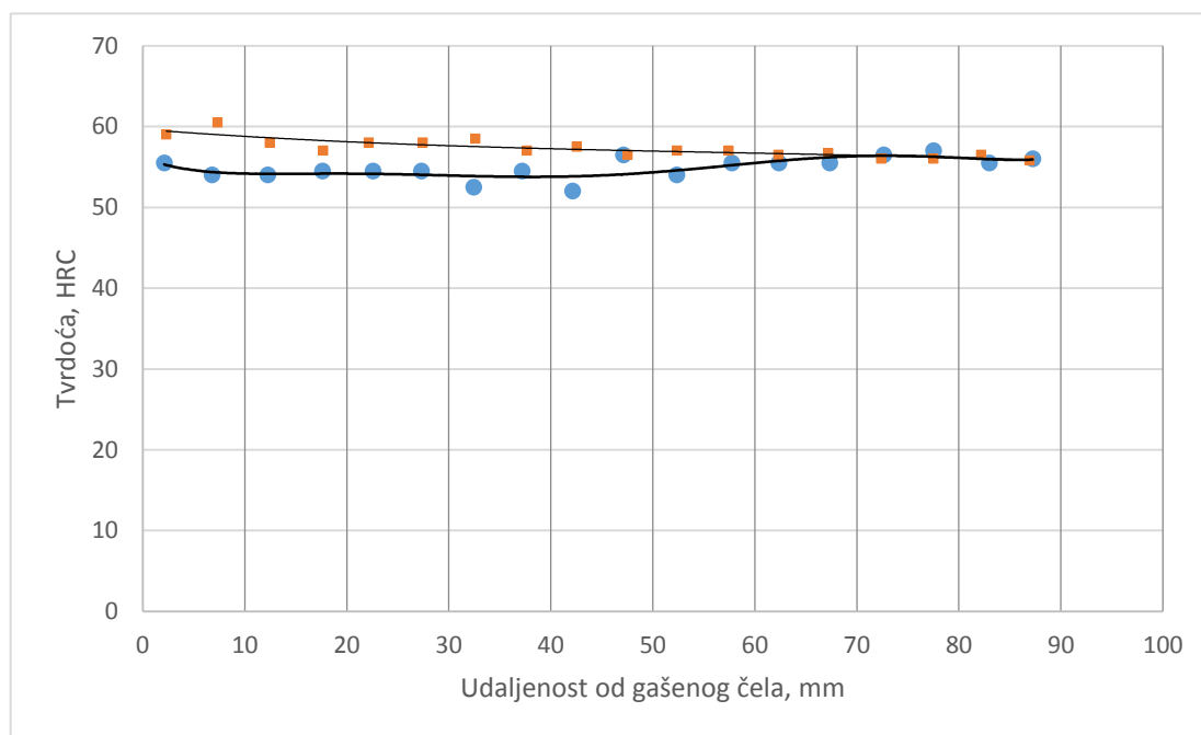
Slika 5.3 Krivulja prokaljivosti epruveta 2 i 3 ohlađenih s temperature 1020°C u izolacijskoj vuni
