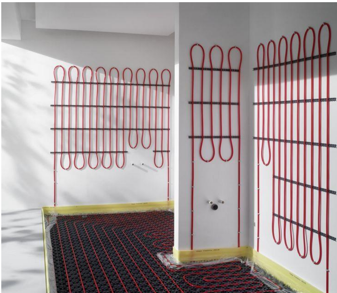
Slika 1.4 Izvedba panelnih grijača
