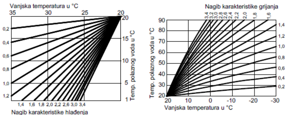
Slika 8.1 Karakteristike grijanja i hlađenja Vitronic 200
