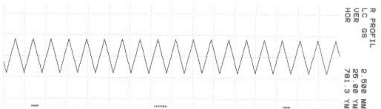
Slika 36. Prikaz simuliranog profila nazivne vrijednosti R_z = 40 \mu\text{m}
